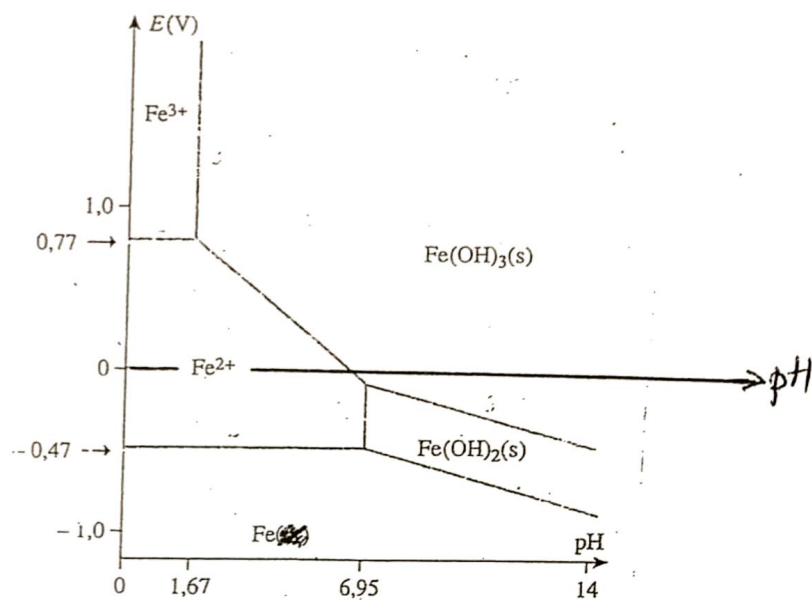
Diagramme E-pH du fer, à 25 °C, pour C_{\text{tra}} = 0,1 \text{ mol} \cdot \text{L}^{-1} .
